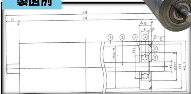
製図例
